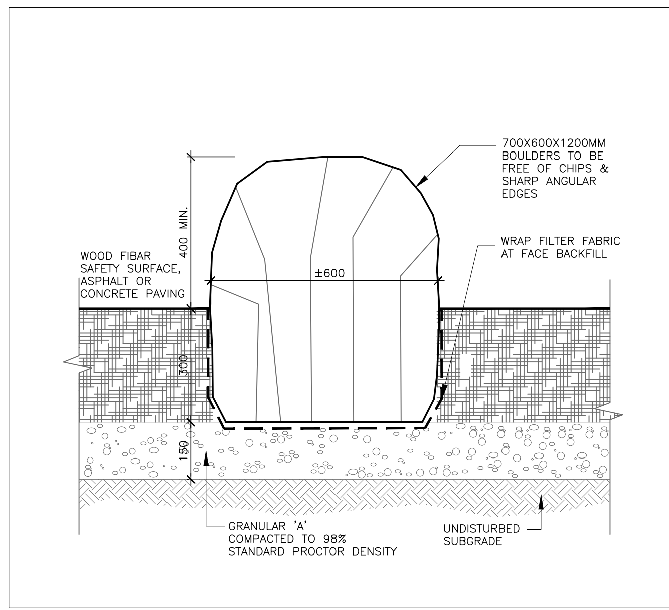
11 BOULDER L-3.0 1:10
