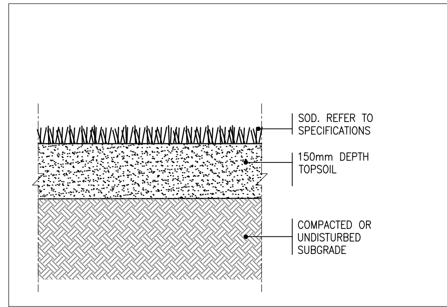
3 SOD L-3.0 1:20
